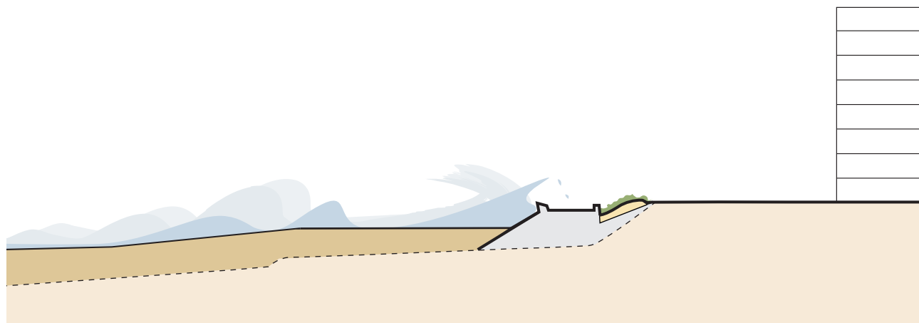
Toekomstige dijk stedelijke zone (40% van de zeedijk) 1,5 km centrum Middelkerke, 500 m centrum Westende
