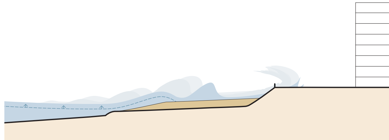
Huidige dijk in geval extreme storm vandaag met suppleties (kunstmatig + vrij grote kosten)
